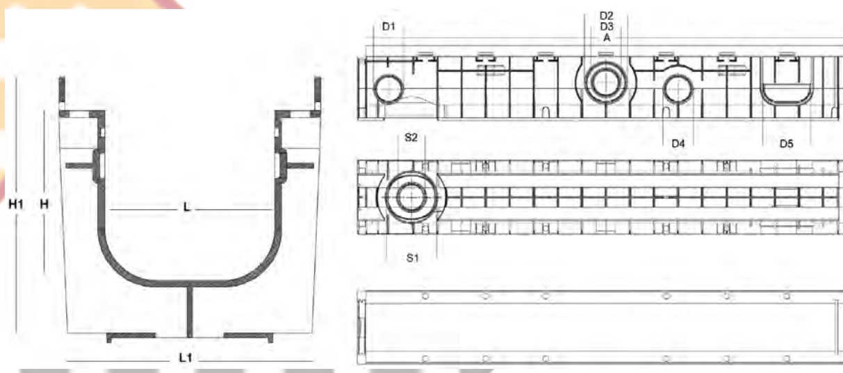
SABDRAIN 601
